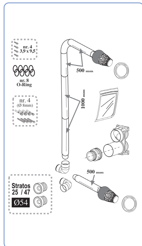
Gescheiden buizenkit in- en uitlaat Ø 54 mm (2 enkelvoudige afsluitstukken)
