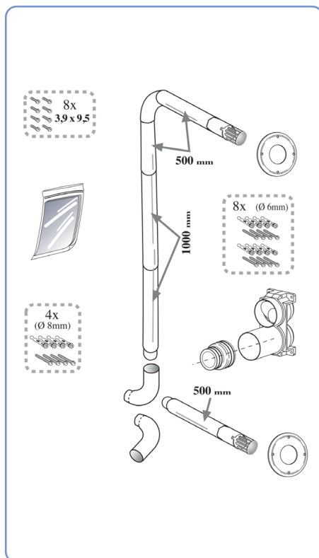
Gescheiden buizenkit in- en uitlaat Ø 32 mm (2 enkelvoudige afsluitstukken)
